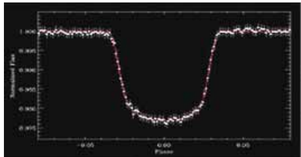
Tránsito del primer exoplaneta observado por COROT (Corot-Exo-1b) © COROT
