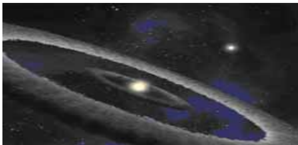
Con la ayuda del telescopio espacial Spitzer de la NASA, los astrónomos han descubierto un cinturón de polvo entorno a la estrella HD 113866 (424AL, 10 Ma) que podría generar un planeta como Marte. © NASA
